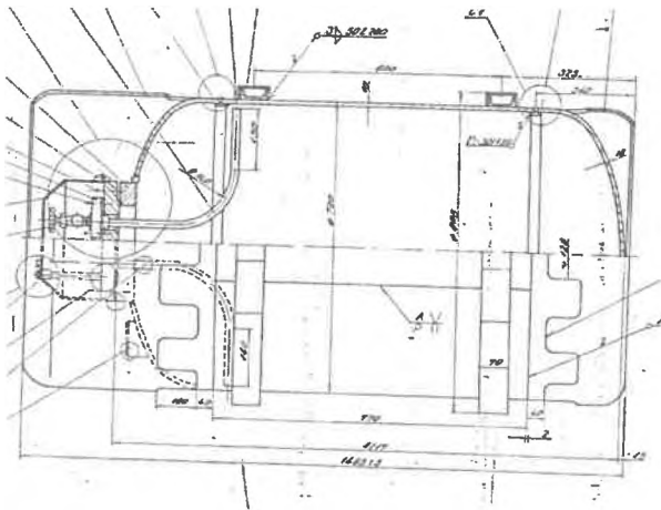
Варел за течен хлор, вместимост 400кг
