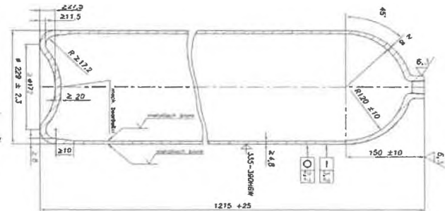
Бутилка за течен хлор, вместимост 40кг
