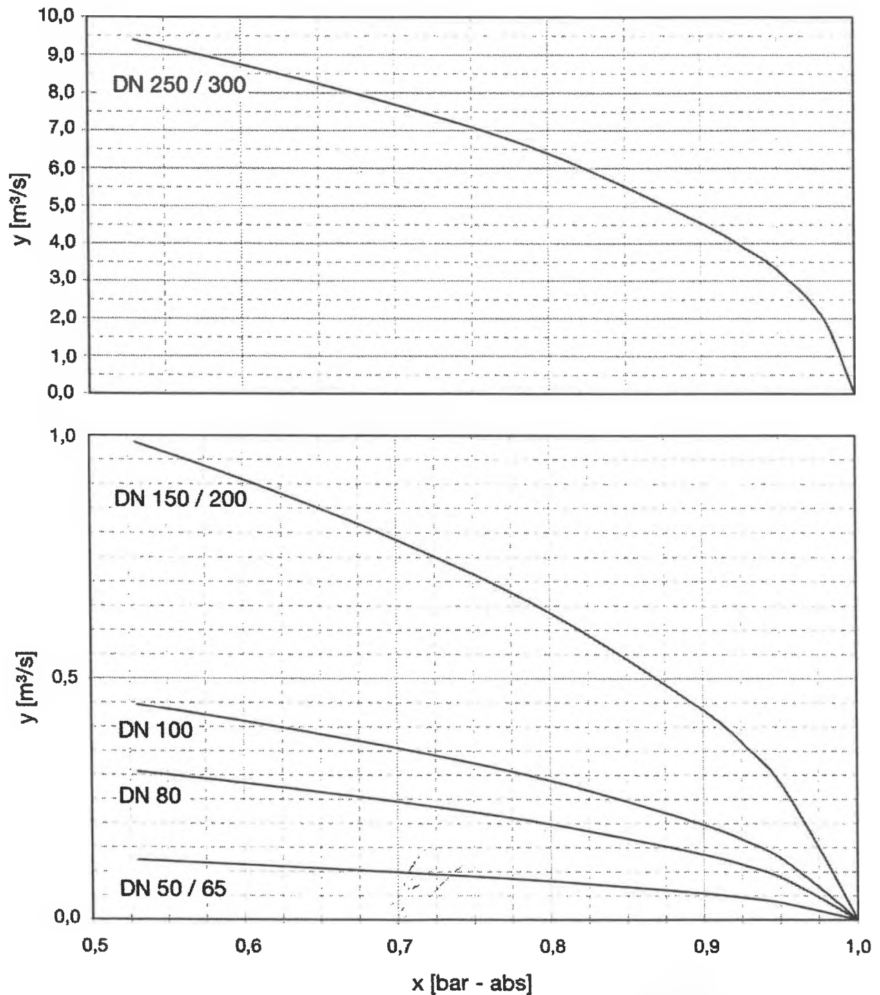
Дебит на всмукване в зависимост от работното налягане Голям отвор
