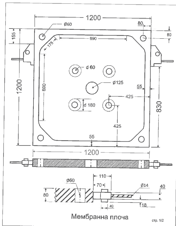
Схема на мембранна плоча на камерни филтър преси Latham 1200
